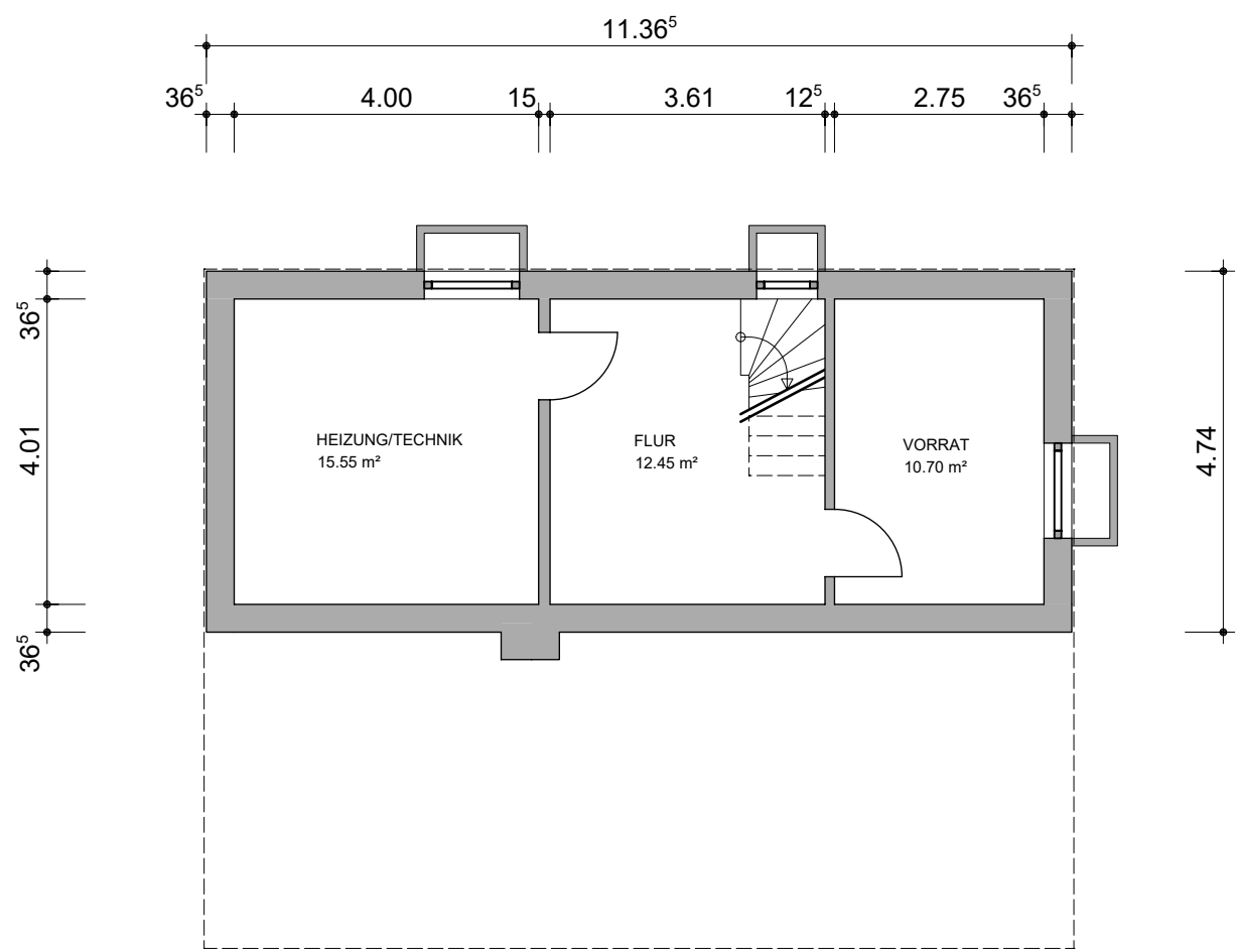
GRUNDRISS KELLERGESCHOSS
