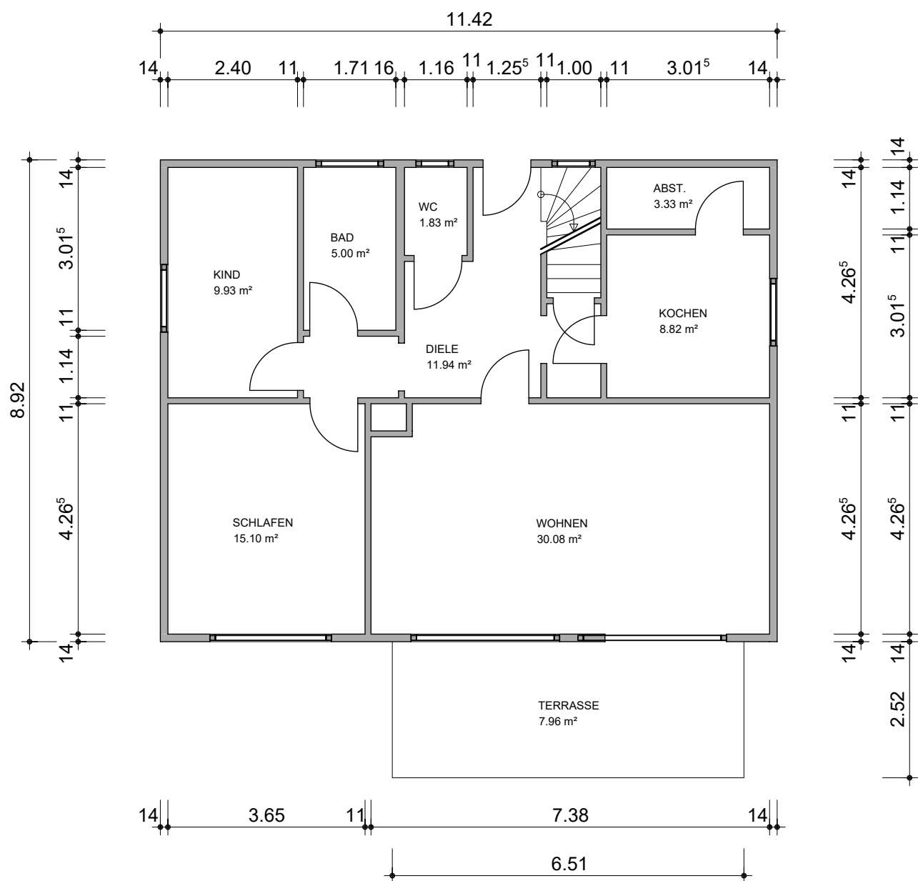
GRUNDRISS ERDGESCHOSS
