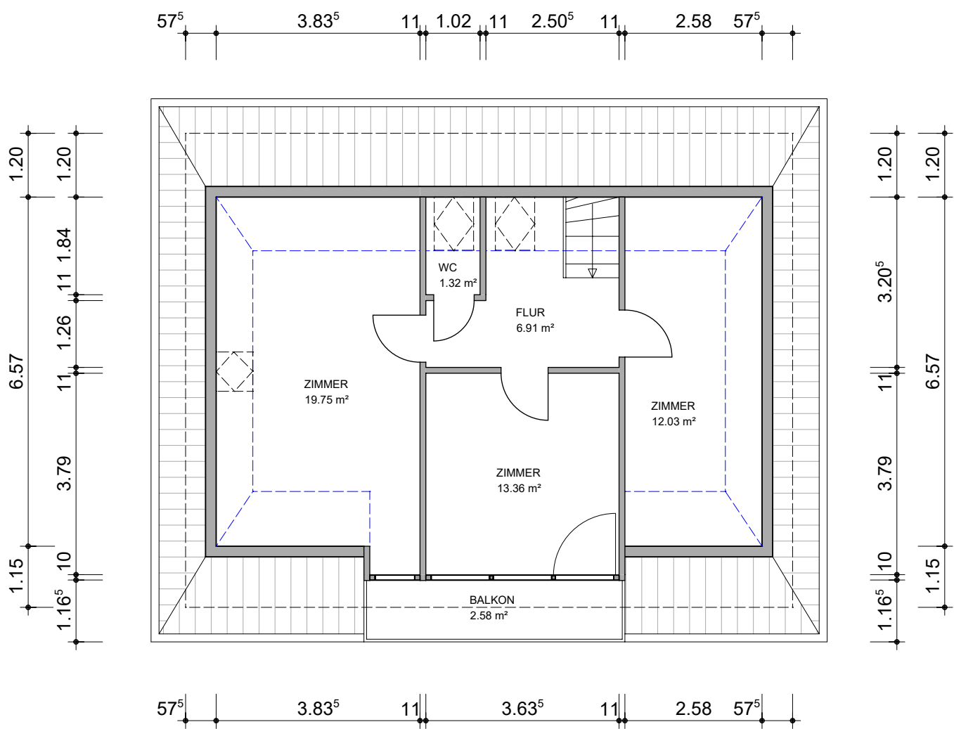
GRUNDRISS DACHGESCHOSS
