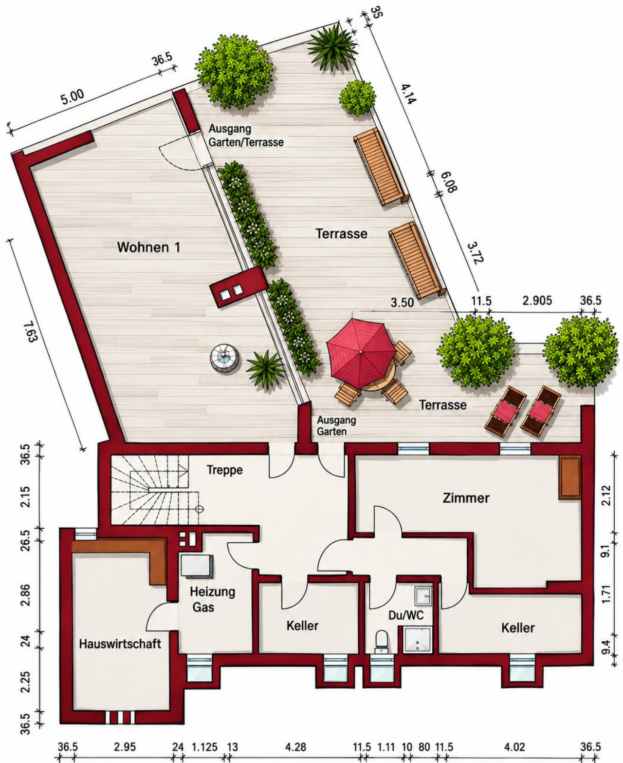
Raumprogramm Ebene Untergeschoss
