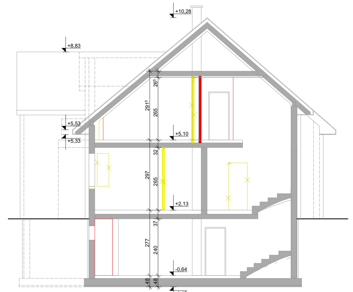
SCHNITT A-A
