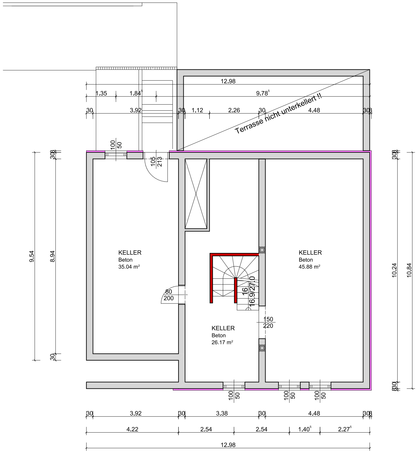
GRUNDRISS KG. 107,09m²
