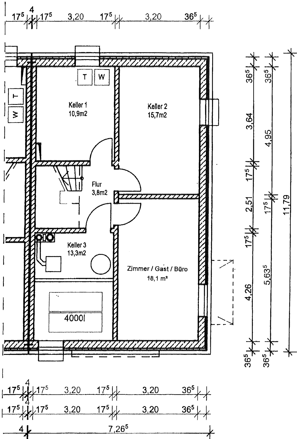
Untergeschoss
