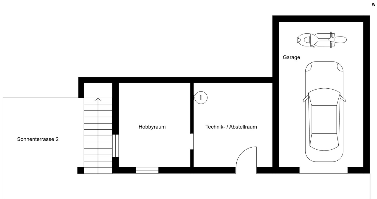
Untergeschoß
