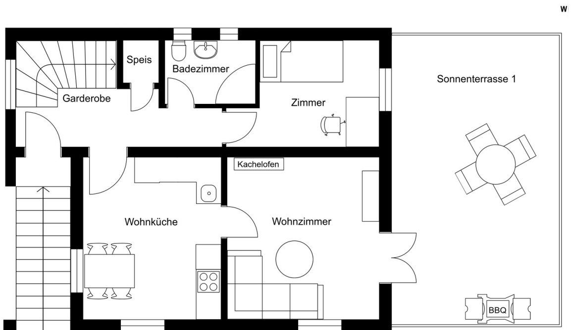
Erdgeschoß
