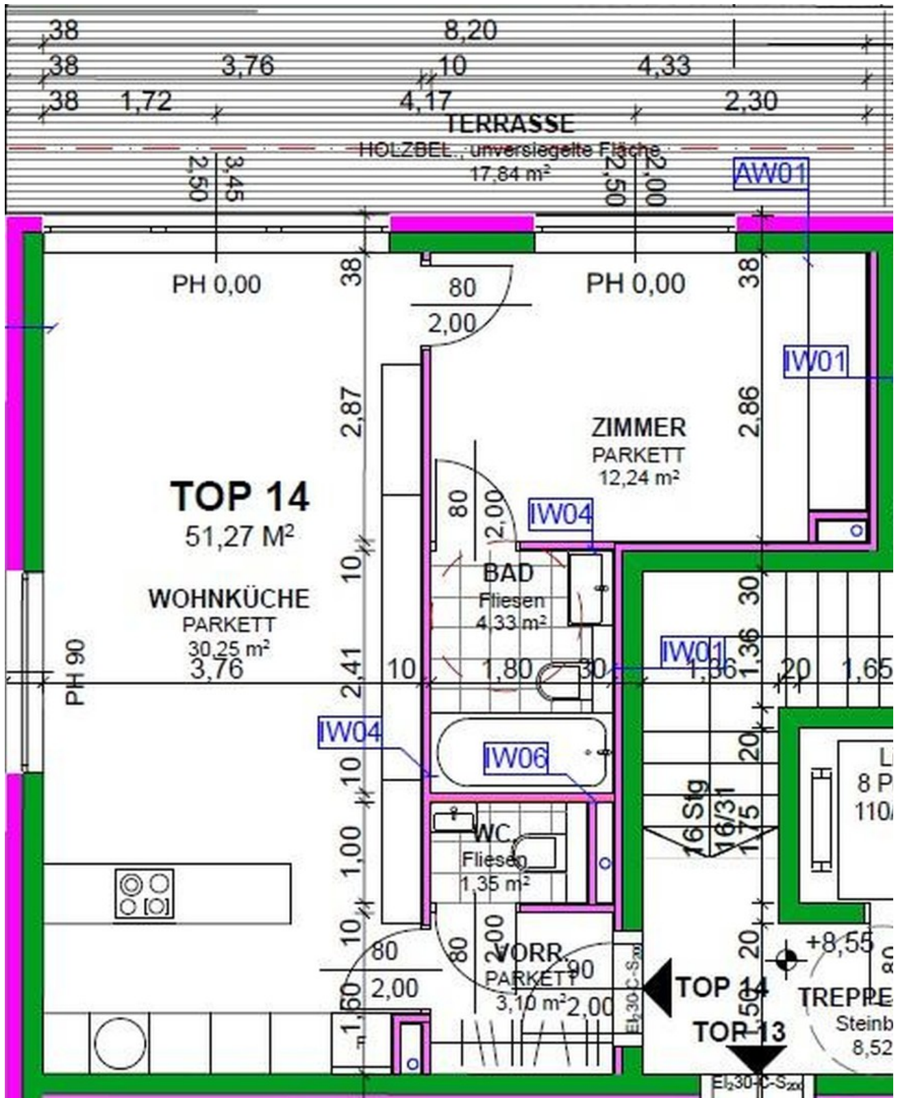
Grundriss - Top 14 - 3.OG
