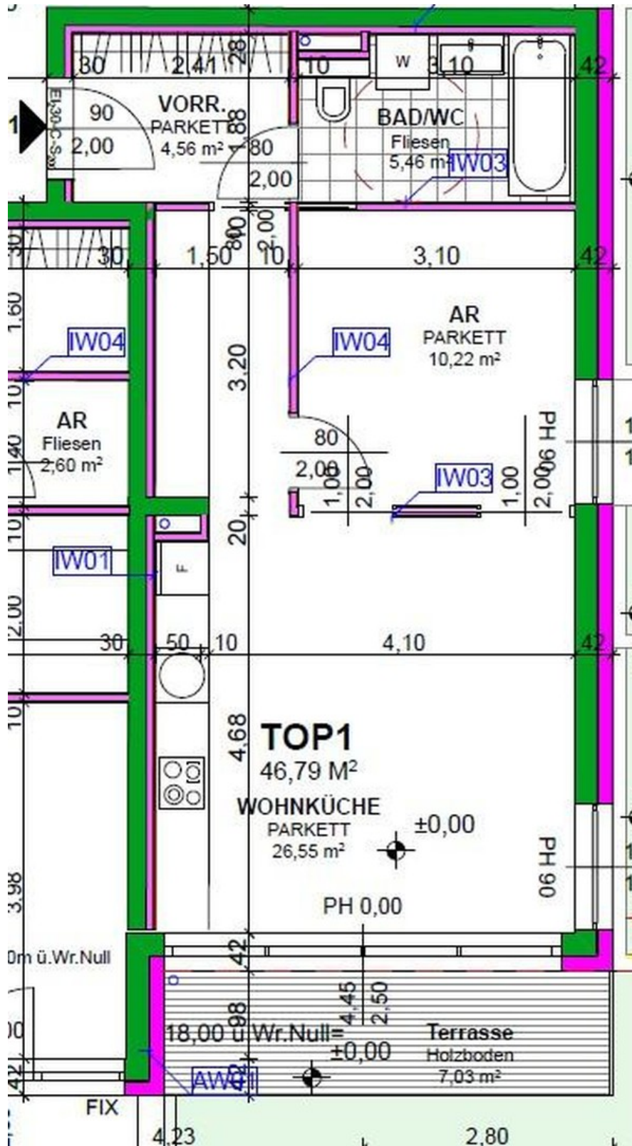
Grundriss - Top 1 - HP
