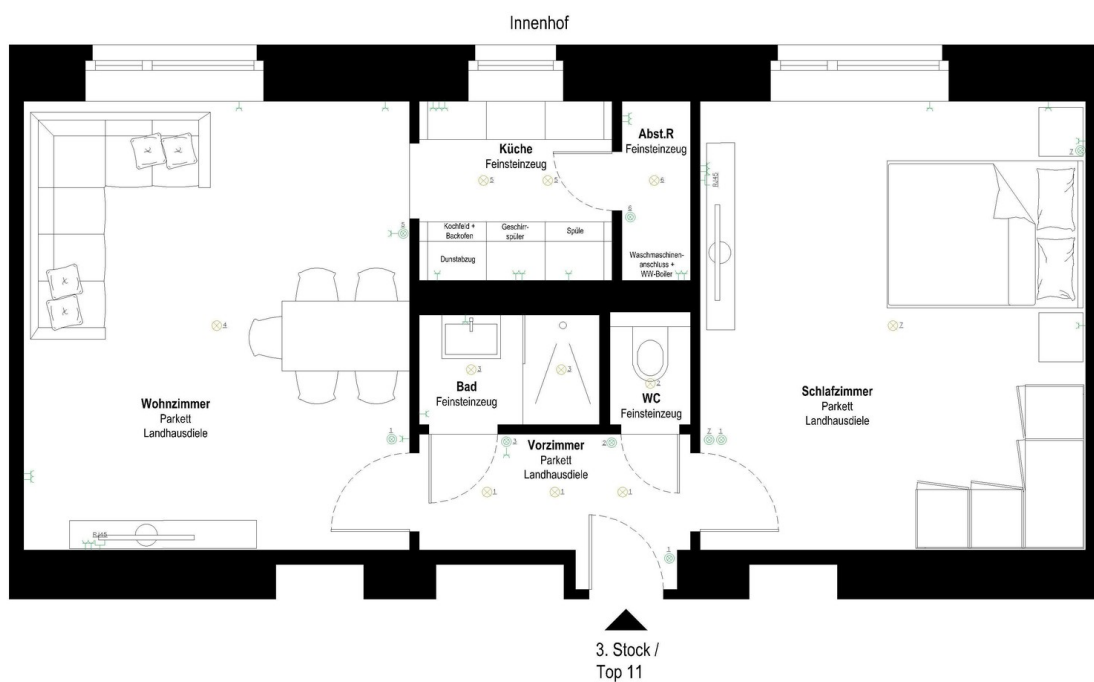
Grundriss
