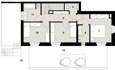
UNTERGESCHOSS MIT GARTEN
