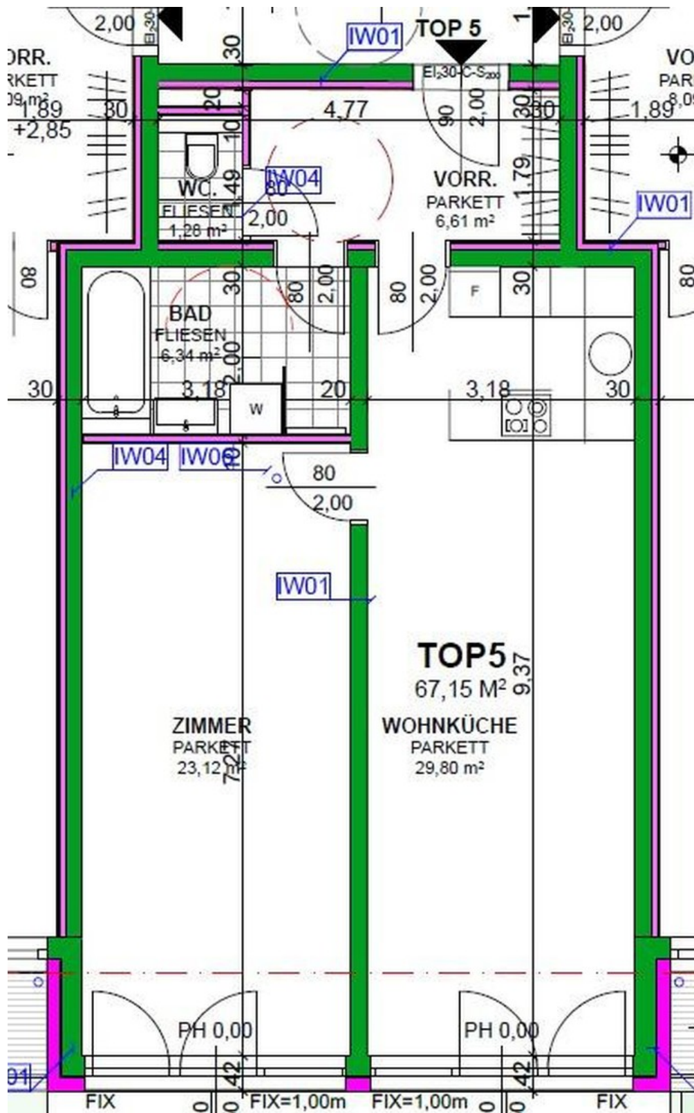
Grundriss - Top 5 - 1. OG
