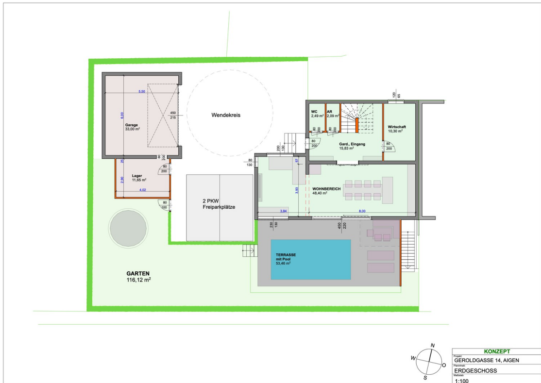
Konzept EG
