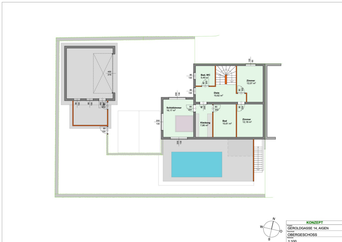
Konzept OG
