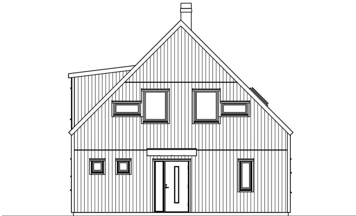
Ansicht Giebelseite Eingang
