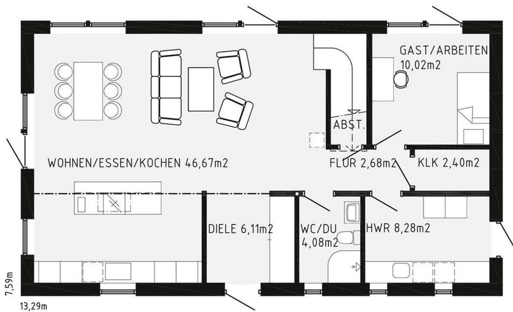
Erdgeschoss (änderbar)
