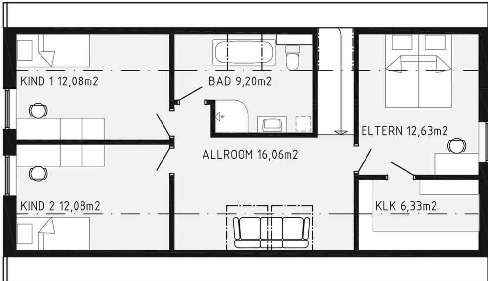
DACHGESCHOSS
