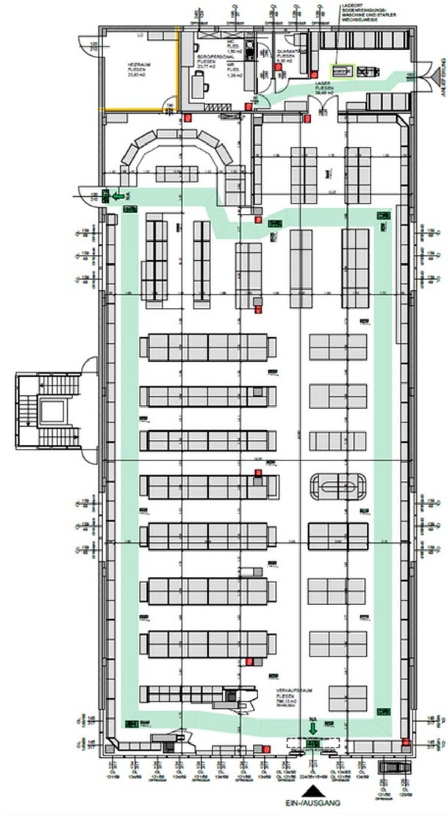
Grundriss EG
