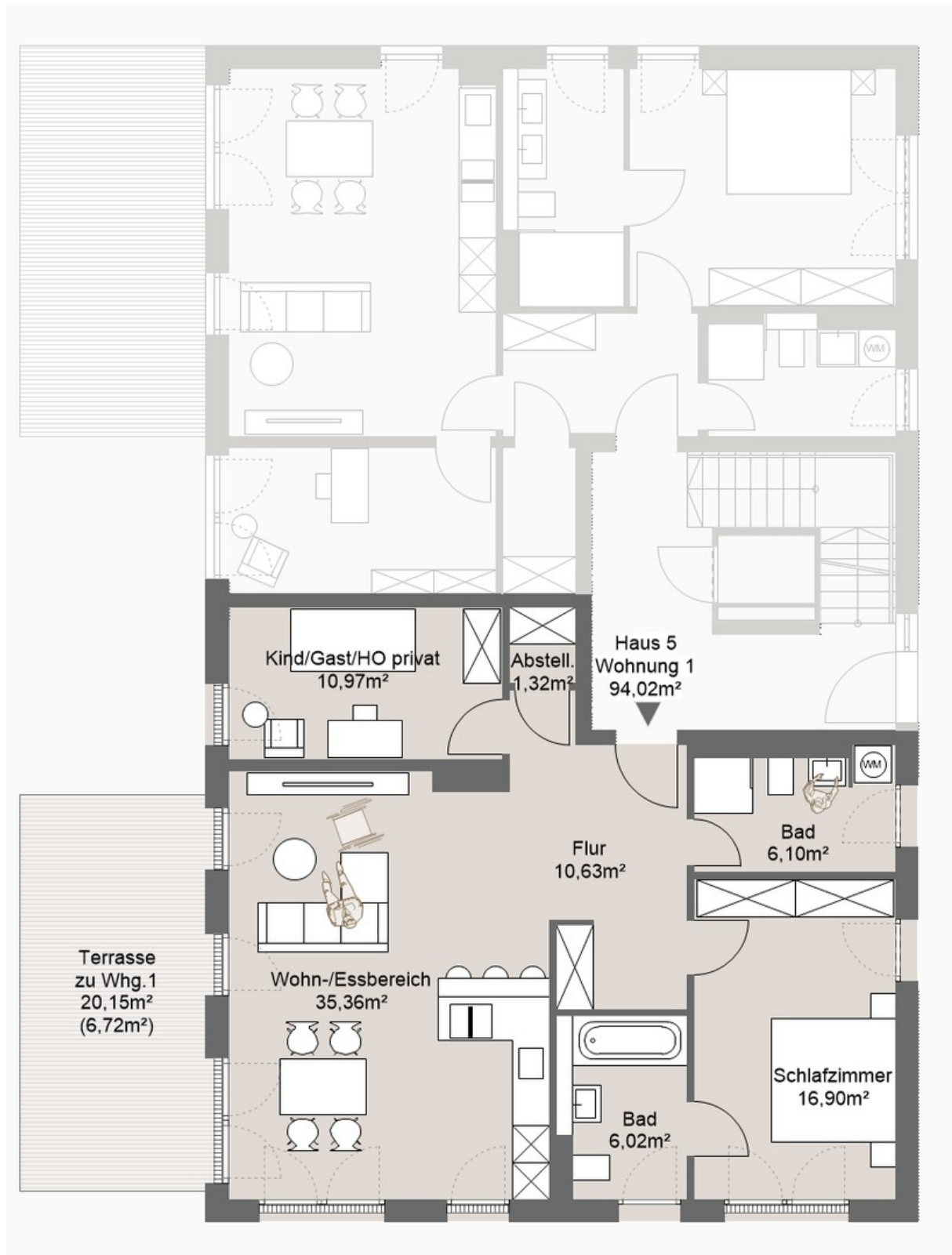
Erdgeschosswohnun Whg. 1
