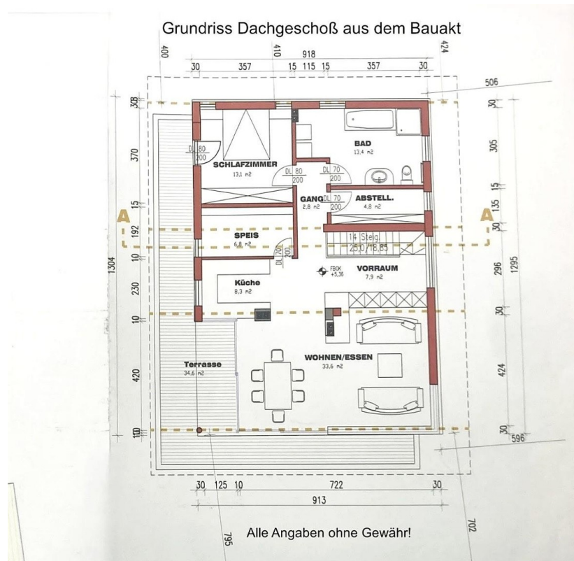
Grundriss Dachgeschoss
