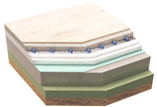
Schema Fußboden Erdgeschoss
