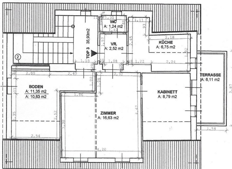
DACHGESCHOSS 1 : 100
