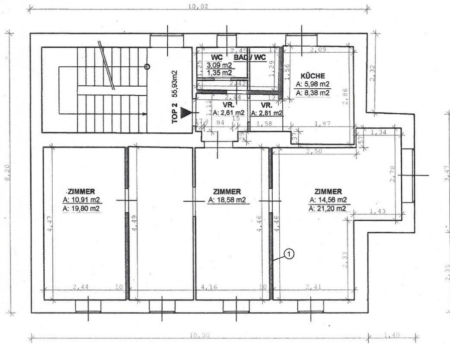
1.STOCK 1 : 100
